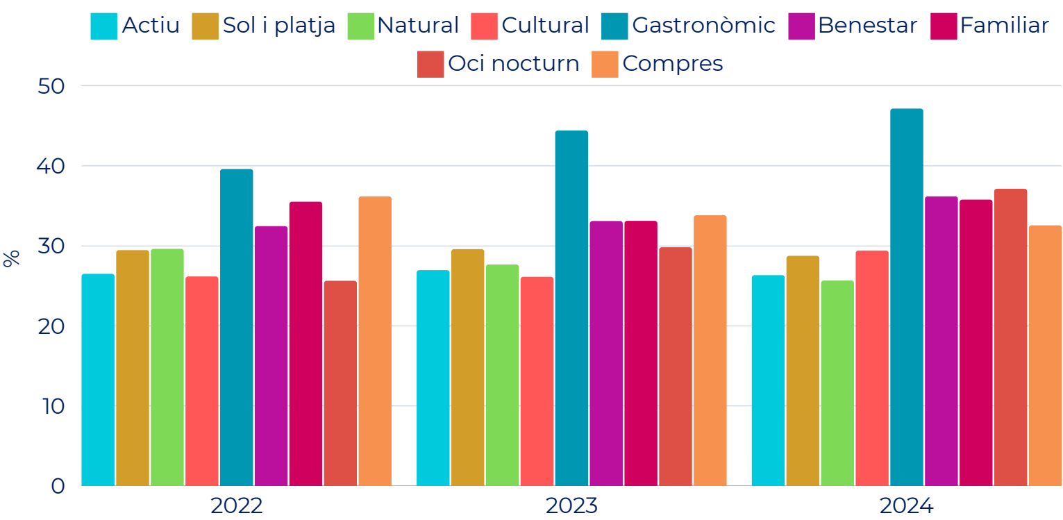
% comentaris positius 2022-2024
